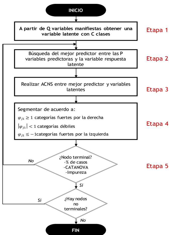
Figura 1. Algoritmo TAID [15]
